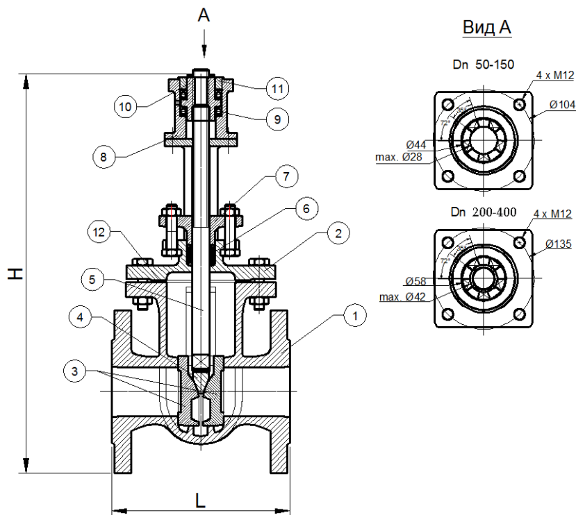
Рис. 1 Конструкция задвижки
